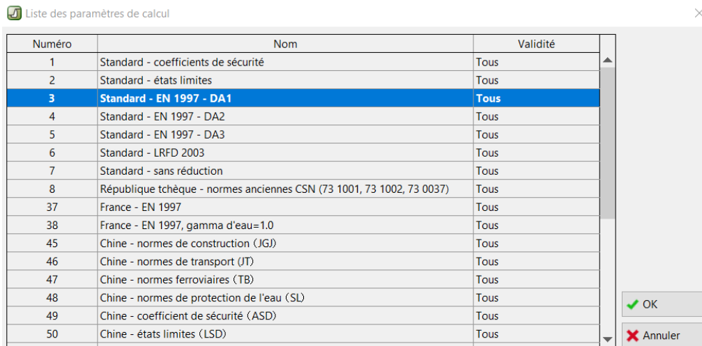
FIGURE 6 – Fenêtre de dialogue « Liste des paramètres de calcul »
