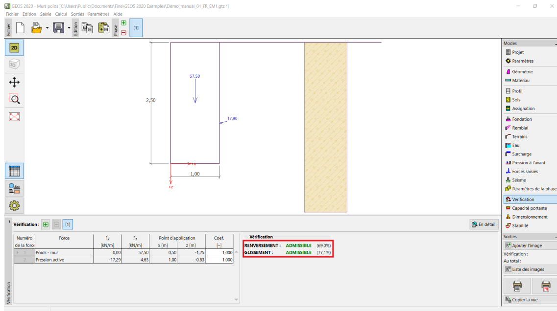
FIGURE 9 – Cadre « Vérification » – Résultats de l'analyse pour SF = 1,6
