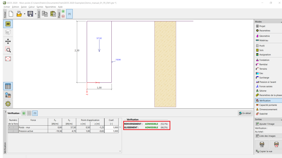
FIGURE 5 – Cadre «Vérification» – Résultats de l'analyse en utilisant la norme CSN 73 0037
