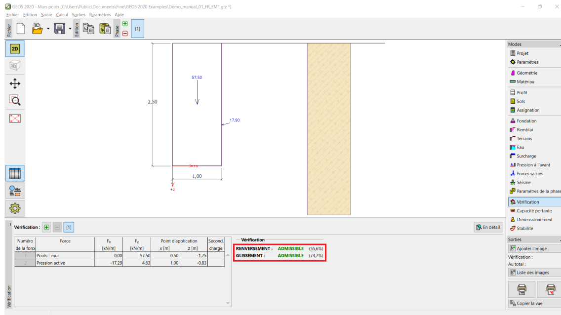
FIGURE 7 – Cadre « Vérification » – Résultats de l'analyse en utilisant la norme EN 1997, DA1
