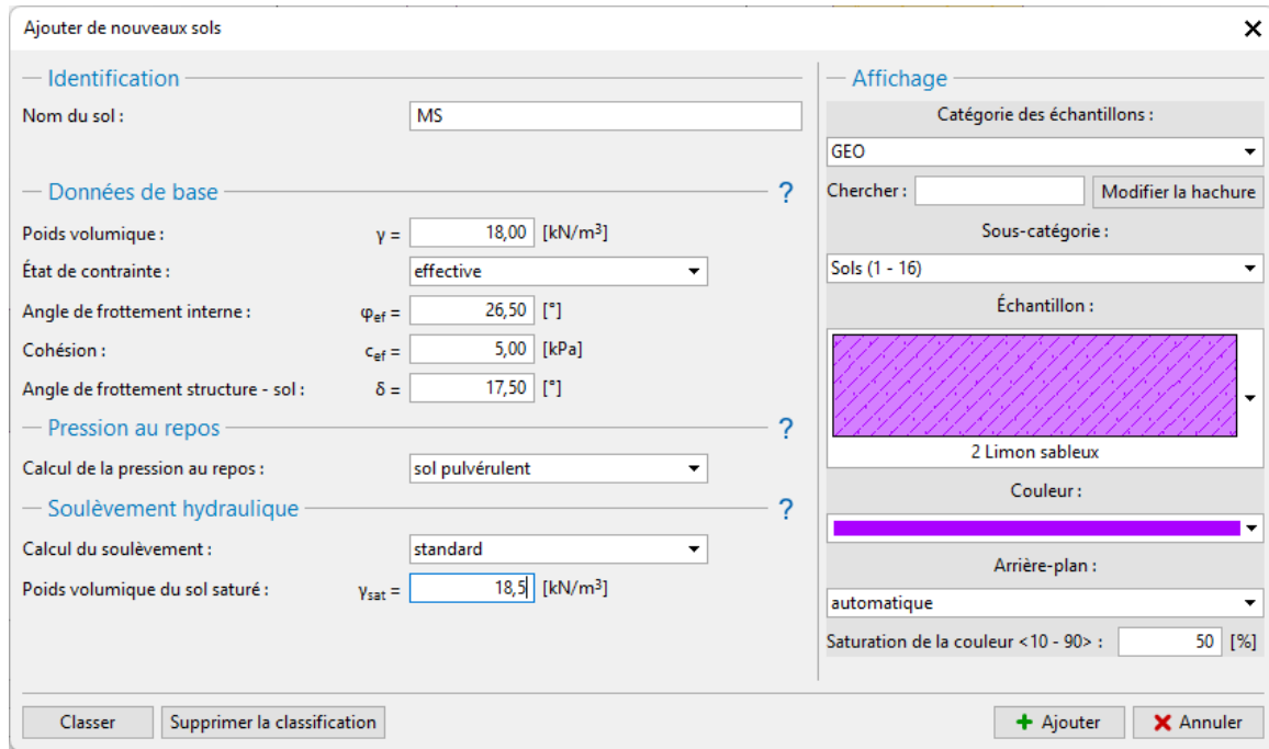
FIGURE 8 – Fenêtre de dialogue « Ajouter des nouveaux sols » - Ajout du sol MS
