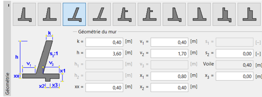
FIGURE 17 – Cadre « Géométrie » - Modification des dimensions du mur cantilever
