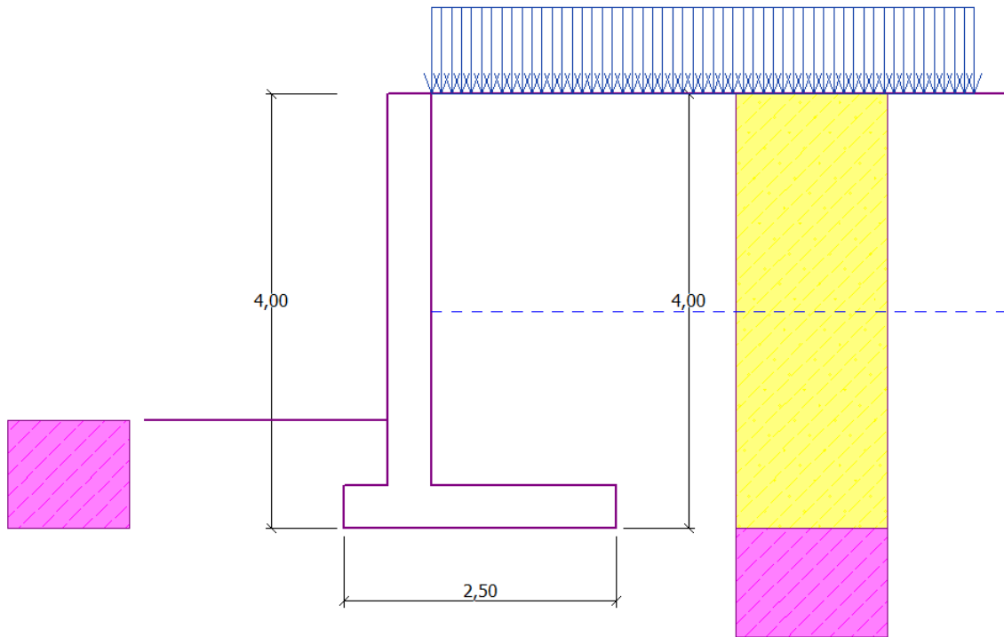
FIGURE 15 – Structure à analyser
