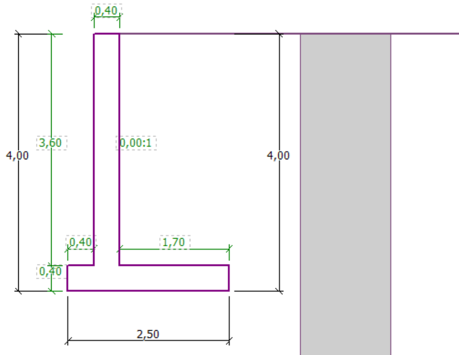
FIGURE 4 – Cadre « Géométrie » - Schéma du mur cantilever
