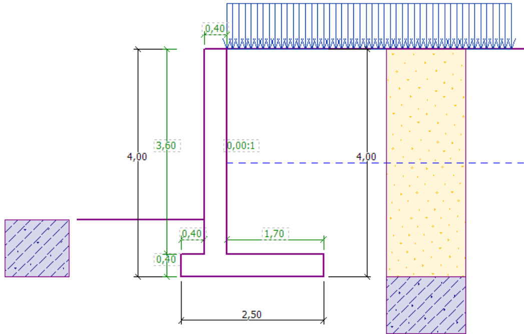
FIGURE 1 – Schéma du mur cantilever – Projet
