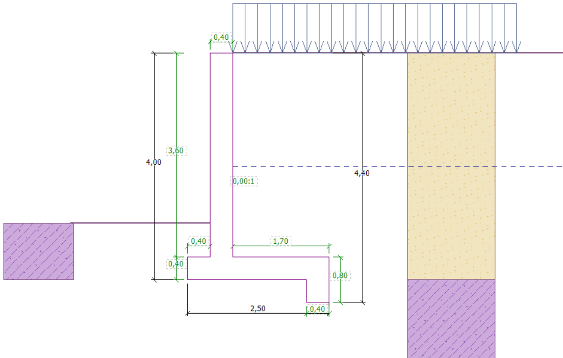
FIGURE 18 – Nouvelle forme de la structure
