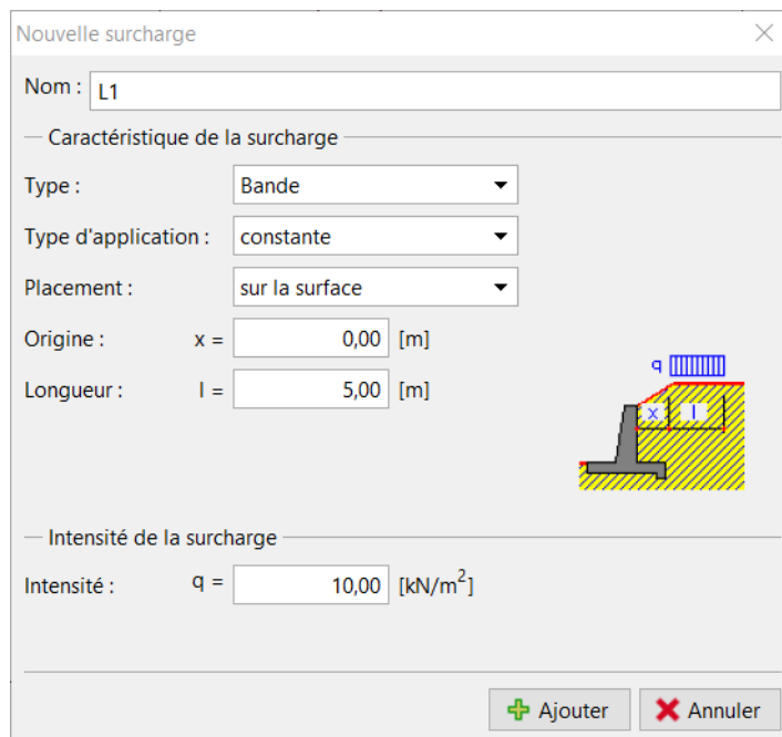
FIGURE 12 – Fenêtre de dialogue « Nouvelle surcharge »
