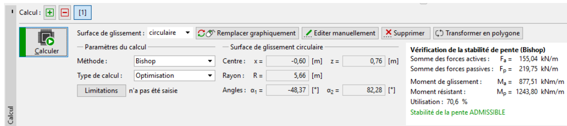
FIGURE 22 – Programme « Stabilité des pentes » - Cadre « Calcul »
